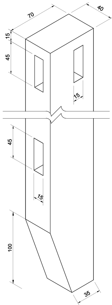
DETAIL A - ขาโต๊ะ = 4 ท่อน
